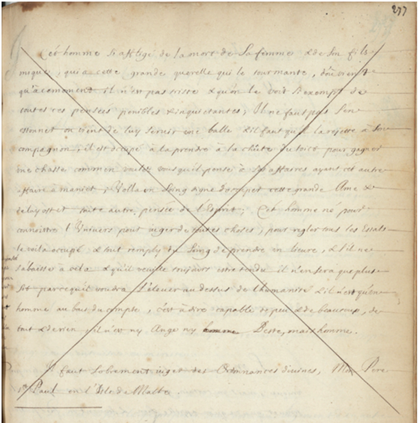
Transcription de C 2 (en rouge : les différences avec C 1 )
